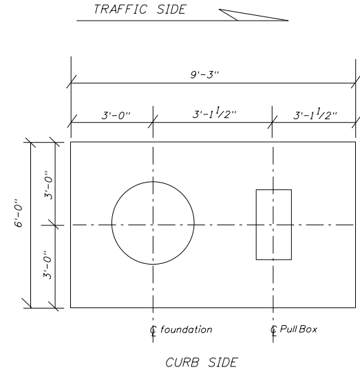
CONCRETE SLAB DETAIL N.T.S.
